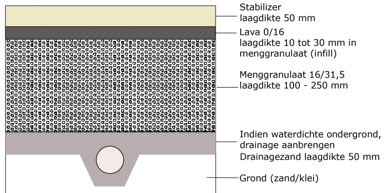
Doorsnede Stabilizer
